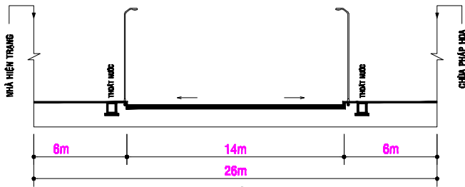
MẶT CẮT (ĐƯỜNG HÀ HOANG HỒ)
