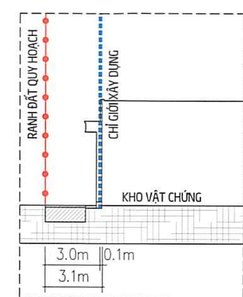
MẶT CẮT 3-3 TỈ LỆ 1/200
