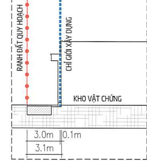
MẶT CẮT 4-4 TỈ LỆ 1/200
