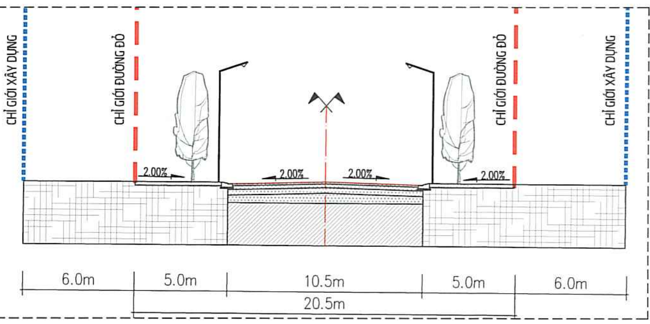
MẶT CẮT A-A TỈ LỆ 1/200
