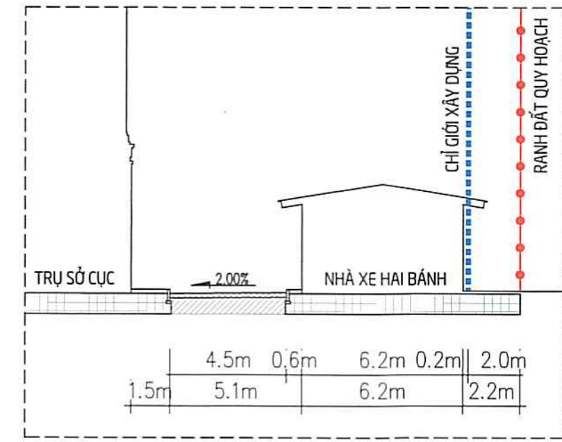
MẶT CẮT 1-1 TỈ LỆ 1/200
